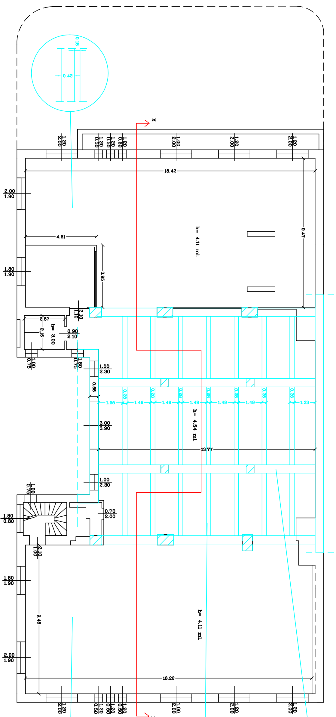
PIANTA PIANO SEMINTERRATO
